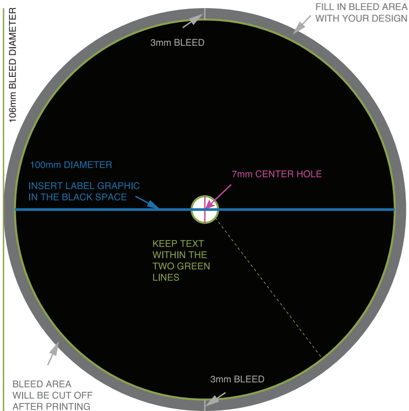
12" LABEL TEMPLATE
